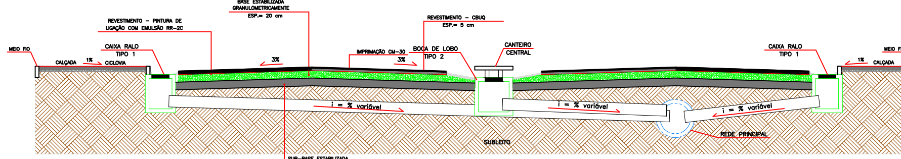
SEÇÃO COM DETALHE DRENAGEM 1/100
