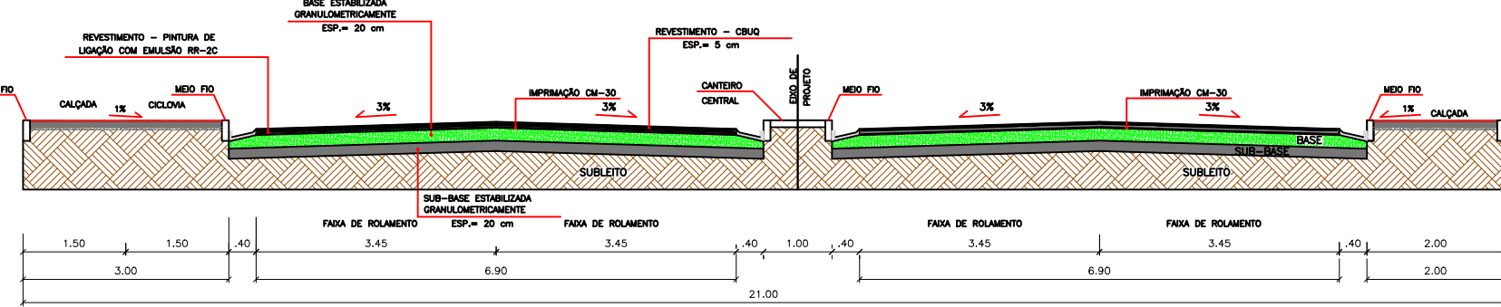
SEÇÃO EM DETALHE CANTEIRO 1/100
