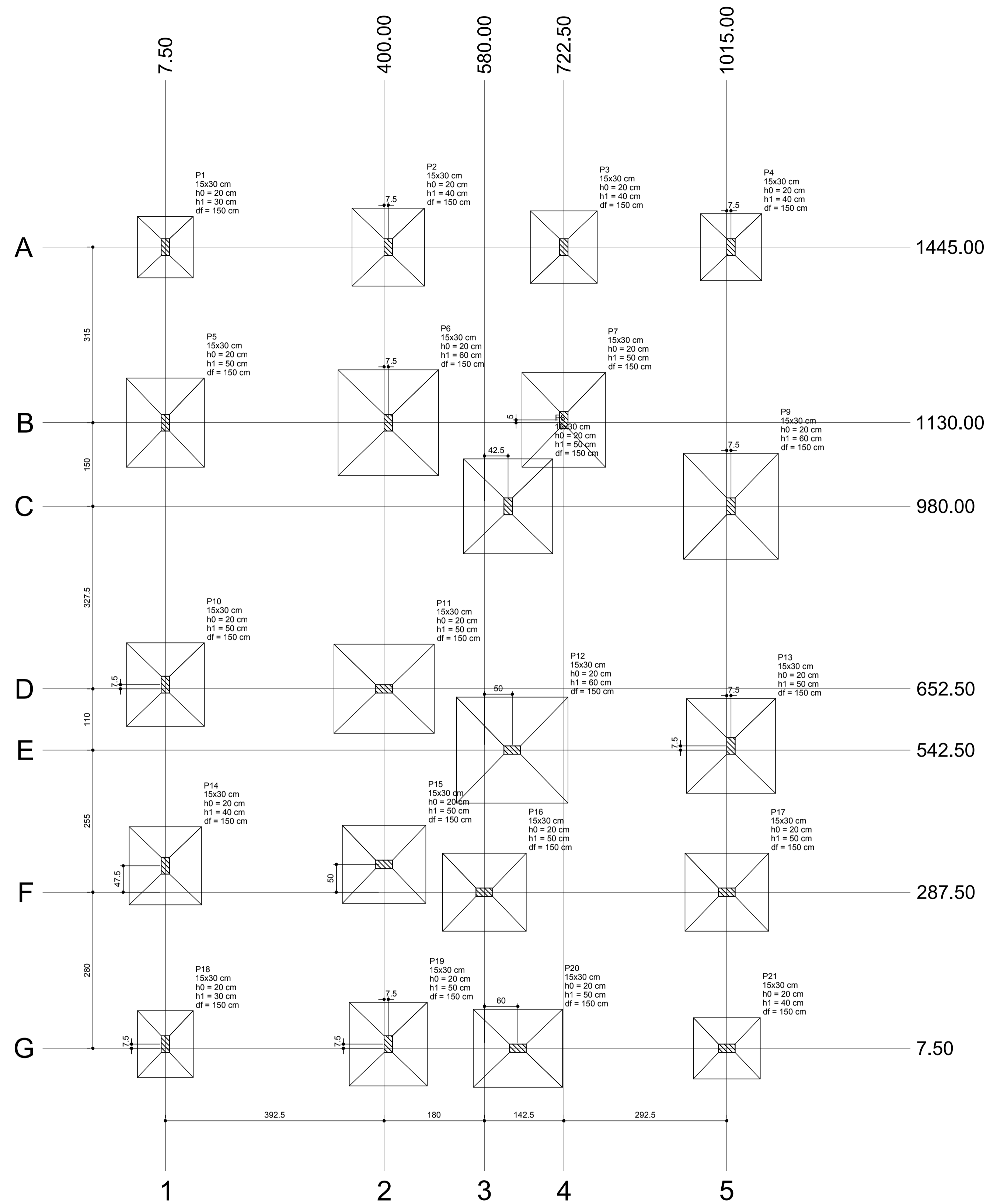
Planta de locação escala 1:50
