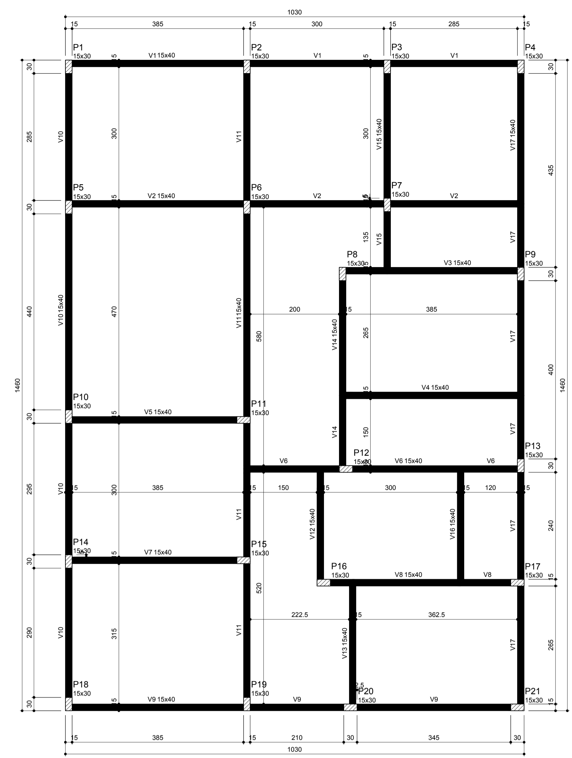
Forma do pavimento FUNDAÇÃO escala 1:50
