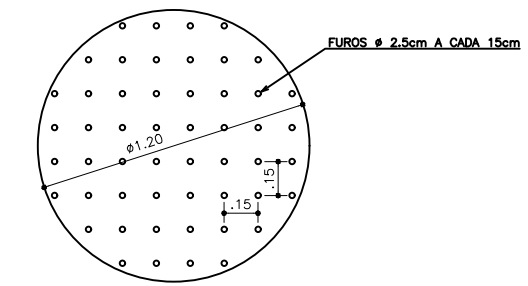
DETALHE - 01 FUNDO FALSO DO FILTRO ANAERÓBIO ESCALA: 1/20
