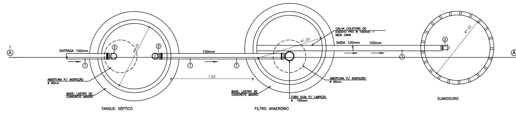
PLANTA BAIXA TANQUE SÉPTICO/FILTRO ANAERÓBIO/SUMIDOURO ESCALA: 1/20
