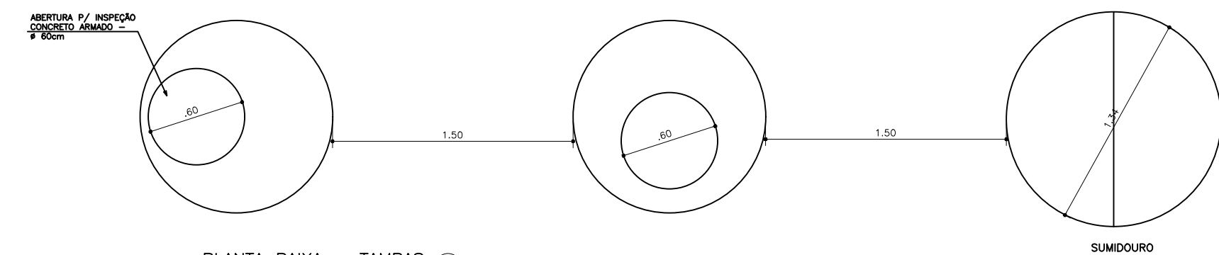
PLANTA BAIXA - TAMPAS TANQUE SÉPTICO/FILTRO ANAERÓBIO /SUMIDOURO ESCALA: 1/20
