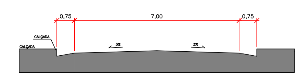
SEÇÃO TIPO 1/100
