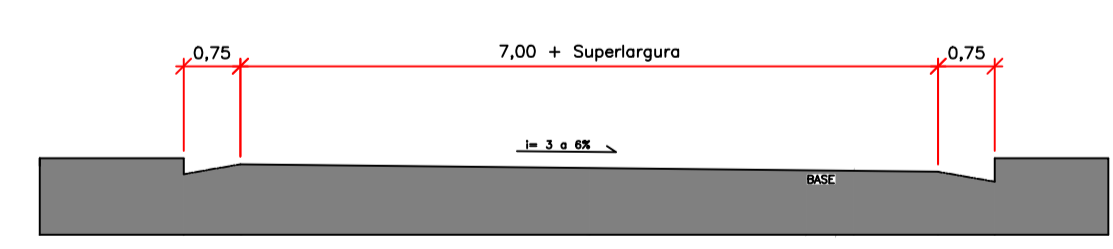
SEÇÃO TIPO – EM CURVA 1/100
